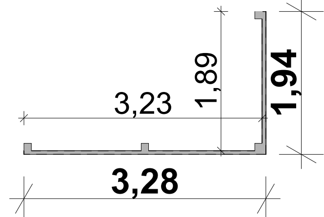
LOCAL POUBELLES - BATIMENT 1 - ECH 1/50
