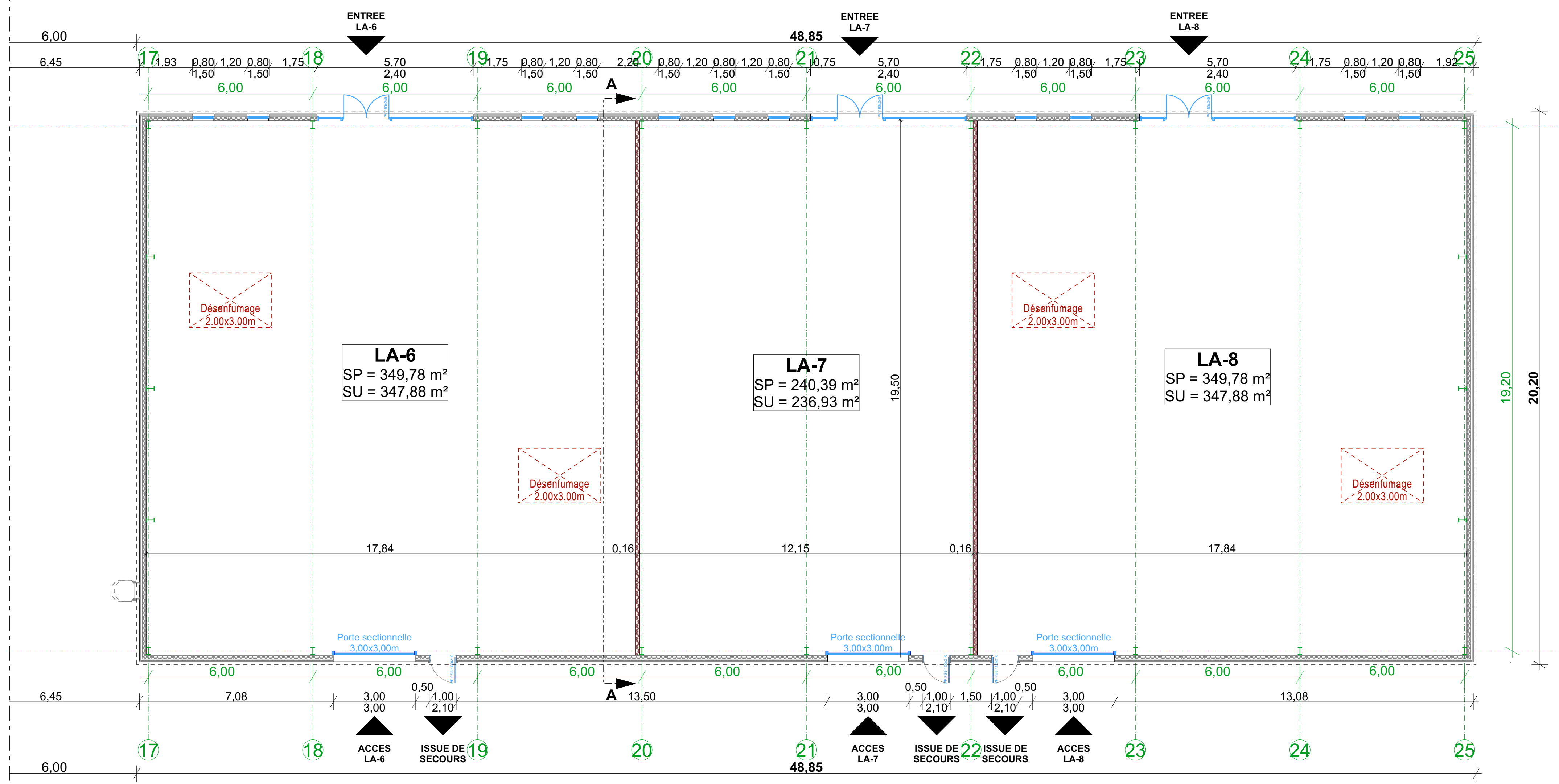
PLAN DU BATIMENT 3
